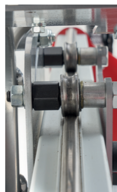
Cuscinetti acciaio che scorrono su doppie barre in acciaio
