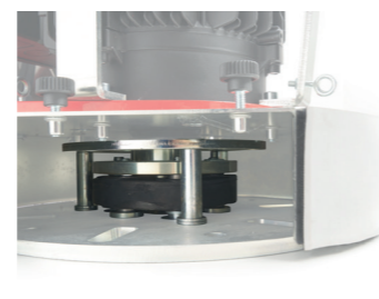
Cuscinetto in gomma per una migliore aderenza al pavimento ed una riduzione delle vibrazioni
