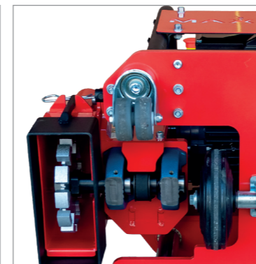
Trasmissione a passo corto con cuscinetti schermati
