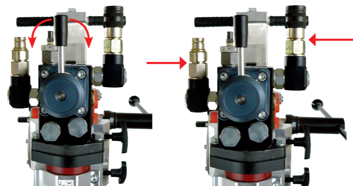
Leva per la regolazione del flusso dell'olio
